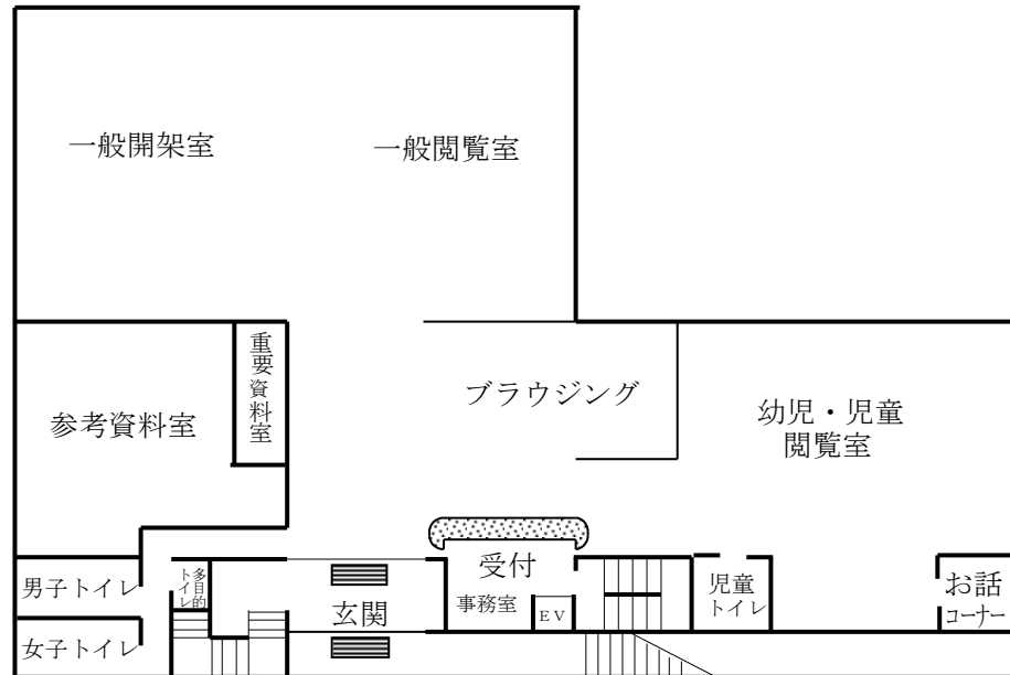
1 階平面図
