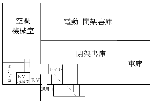
地階平面図
